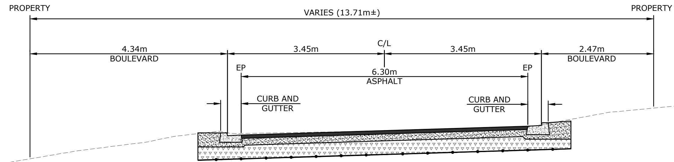
A-A 001A SCALE: 1:50 TYPICAL SECTION STA. 0+020 TO 0+060
