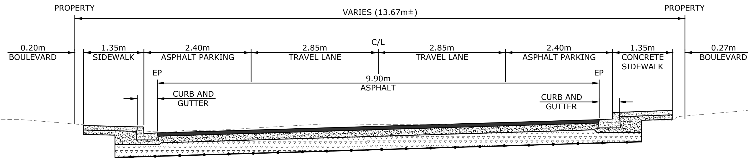
B-B 001A SCALE: 1:50 TYPICAL SECTION STA. 0+075 TO 0+150
